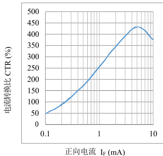
图.2 电流转换比 vs. 正向电流曲线图
