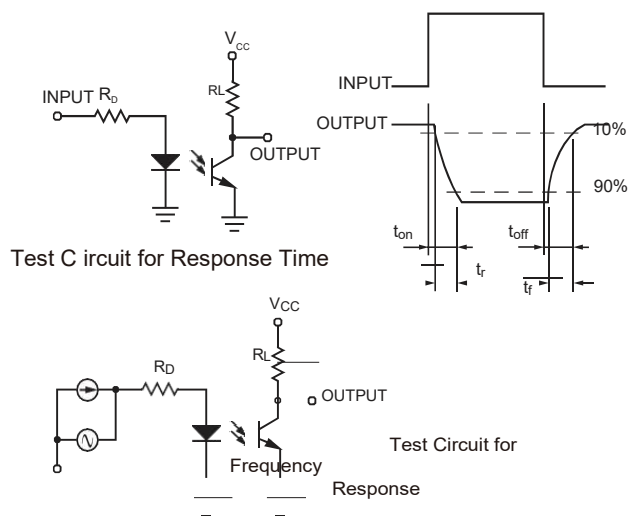
图.1测试电路
